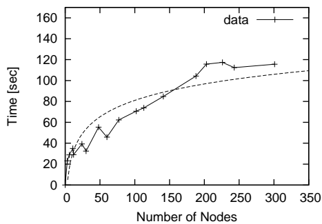
図 11 バンド幅マップ構築にかかる時間
